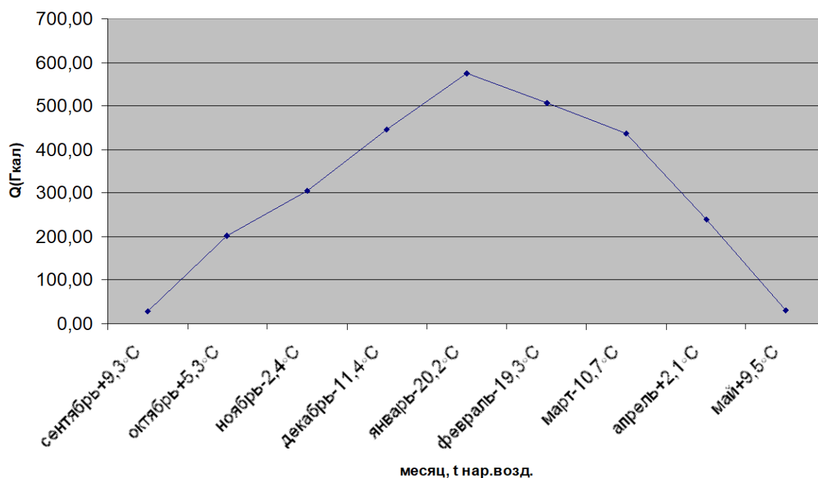
График годовых тепловых нагрузок по котельной с.Кавказское
