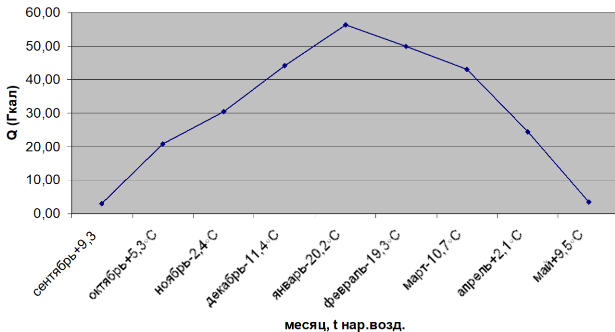
График годовых тепловых нагрузок по котельной с. Знаменка ЦРБ
