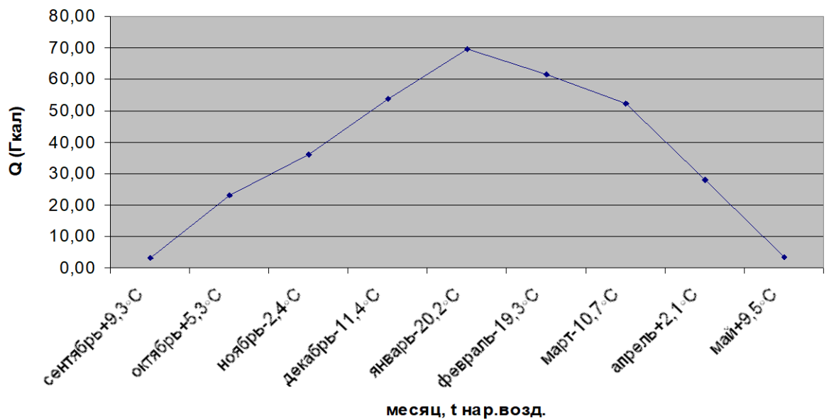
График годовых тепловых нагрузок по котельной с. Восточное
