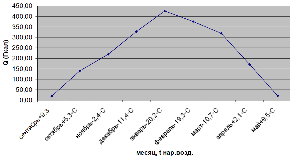
График годовых тепловых нагрузок по котельной с. Знаменка школа
