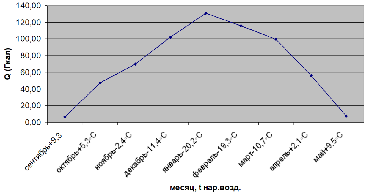
График годовых тепловых нагрузок котельной с. Верхняя Коя
